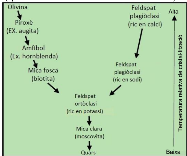
Sèries de reacció de Bowen
