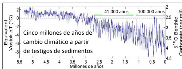
Cambios de temperatura en los últimos 5 millones de años, según las proporciones de ^{18}\text{O}:^{16}\text{O} en las conchas de microorganismos de sedimentos profundos – frío hacia abajo, calor hacia arriba.
